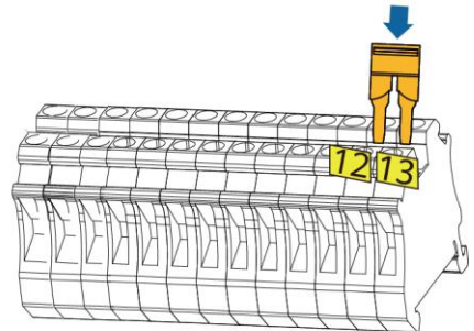
Borne de CA del inversor X3 (trifásico)
