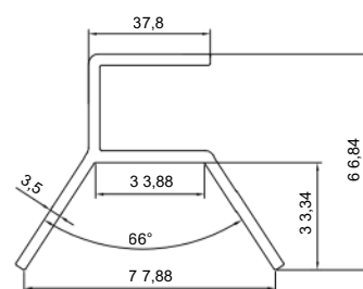
Medidas
