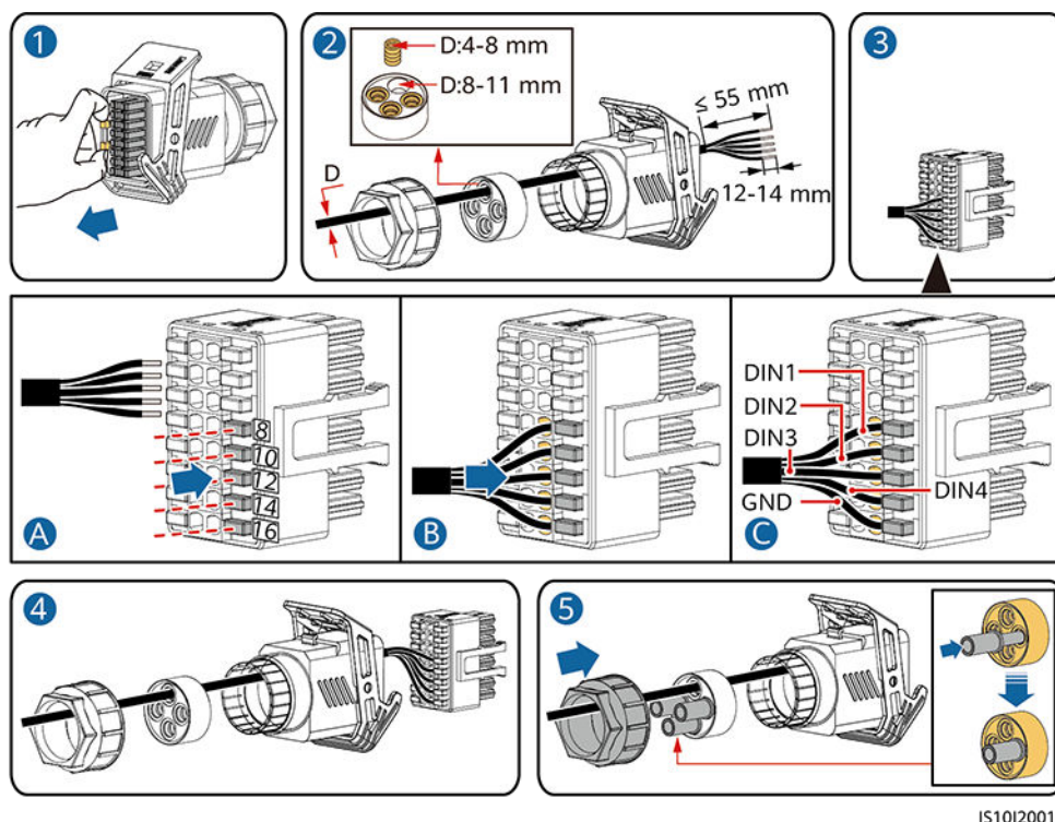
Figura 5-42 Instalación del cable
