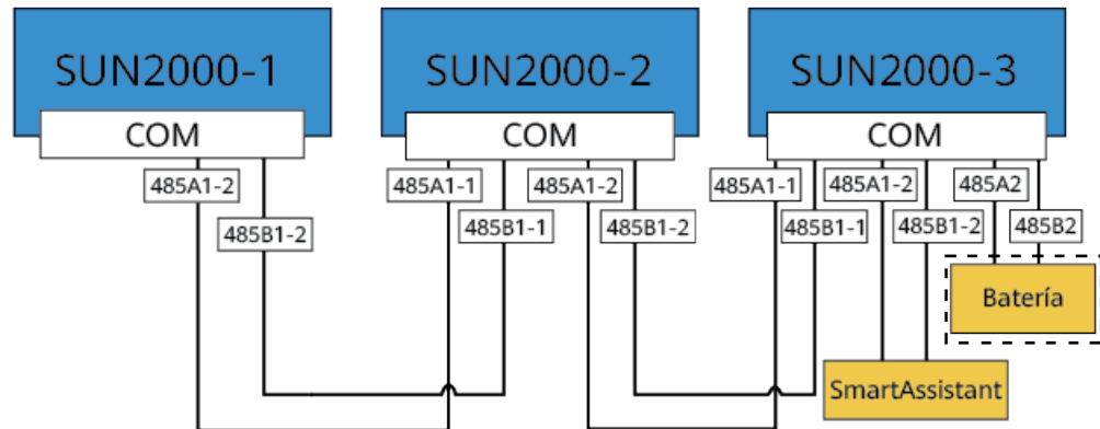
Figura 5-23 Conexión en red del SmartAssistant (los componentes opcionales están encerrados en cuadros de rayas pequeñas)
