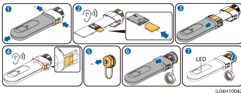
Figura 5-18 Instalación del Smart Dongle 4G (SDongleB-06)
