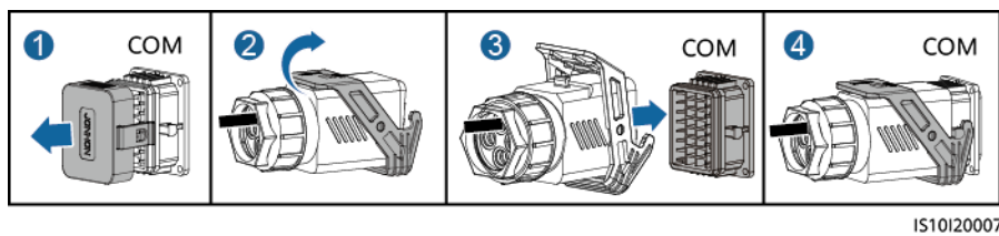
Figura 5-45 Fijación del conector del cable de señal
