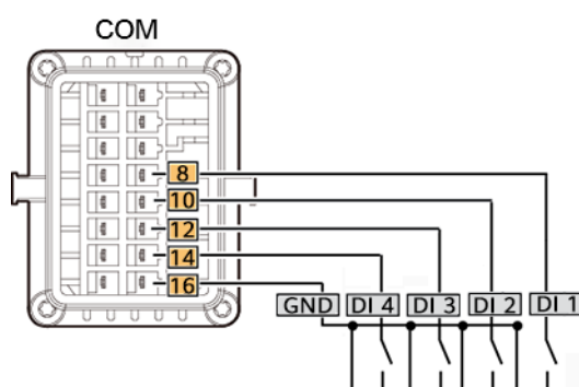
Figura 5-40 Conexiones de los cables (conexión a red del Smart Dongle, el SmartAssistant y el Smart Guard)
