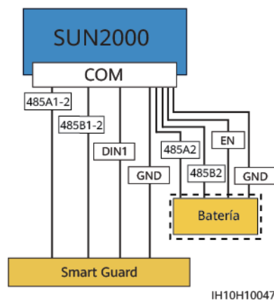
Figura 5-24 Conexión en red del Smart Guard (los componentes opcionales están encerrados en cuadros de rayas pequeñas)
