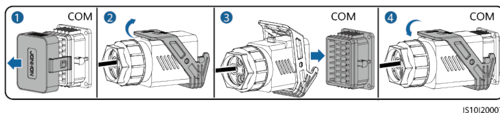
Figura 5-43 Fijación del conector del cable de señal
