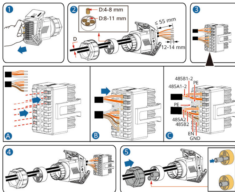
Figura 5-36 Instalación de los cables
