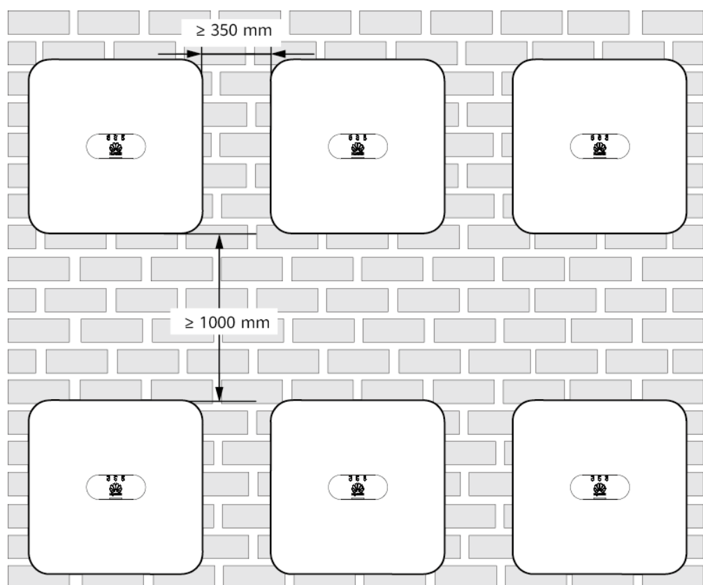
Figura 4-5 Instalación apilada (no recomendada)
