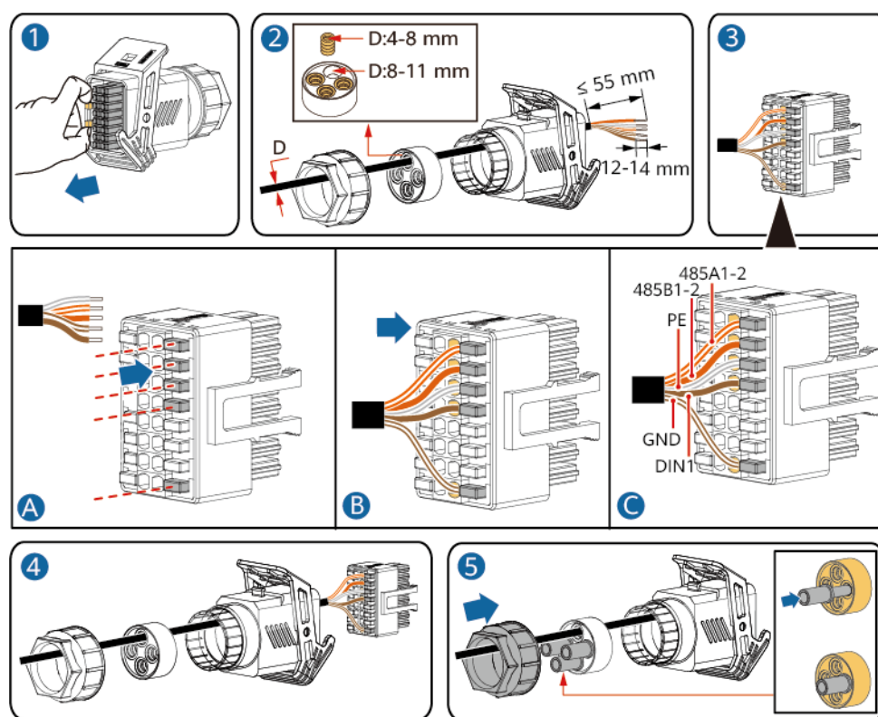
Figura 5-38 Instalación del cable
