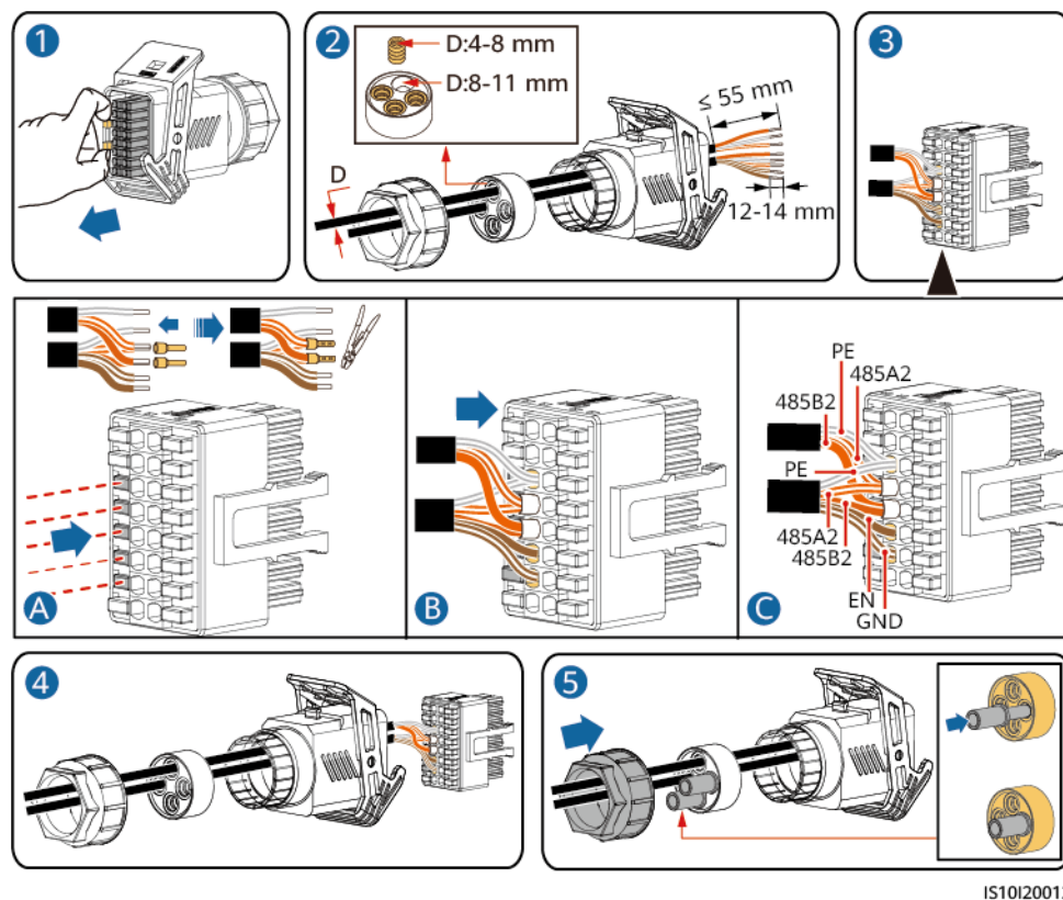
Figura 5-32 Instalación del cable
