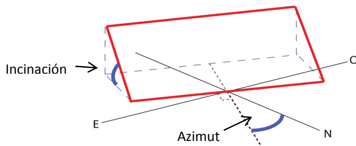
Figura 3: Esquema de un panel solar donde se señalan los ángulos de inclinación y azimut que definen su posición.
