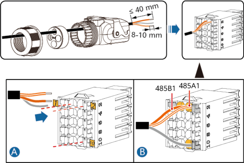
Figura 5-22 Instalación del cable (conexión al SmartAssistant)
