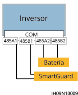
Figura 5-16 Conexión a red del SmartGuard
