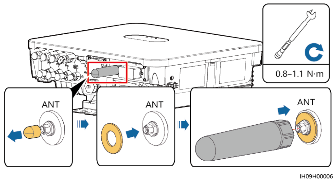
Figura 5-39 Instalación de una antena WLAN
