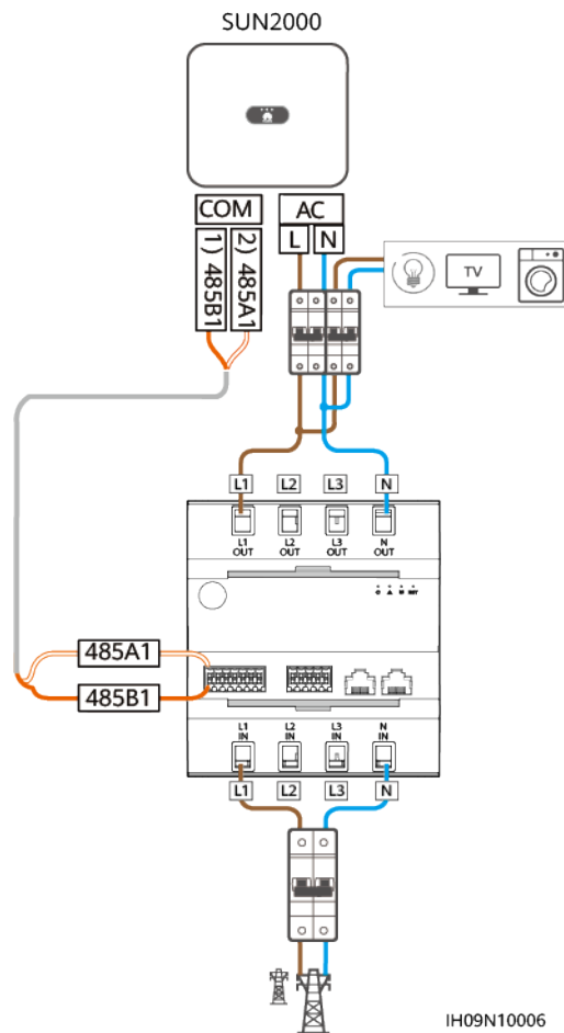
Figura 5-21 Conexión de los cables al SmartAssistant
