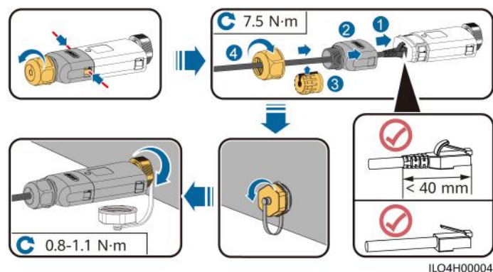
Figura 5-35 Instalación del Smart Dongle WLAN-FE (comunicación FE)
