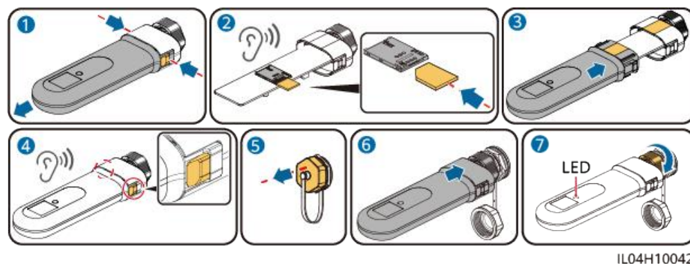
Figura 5-37 Instalación del Smart Dongle 4G (SDongleB-06)
