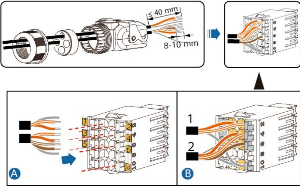
Figura 5-23 Instalación de los cables (conexión al SmartAssistant y a la batería)
