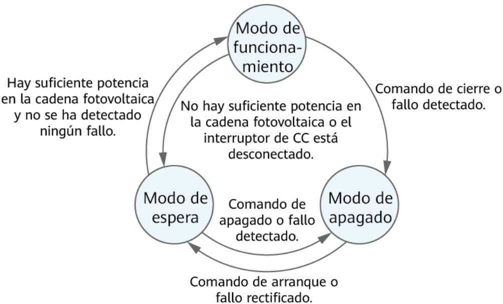
Figura 2-7 modos de operación
