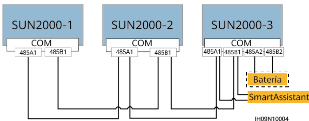
Figura 5-15 Conexión a red del SmartAssistant (el componente encerrado en el cuadro de rayas pequeñas es opcional)
