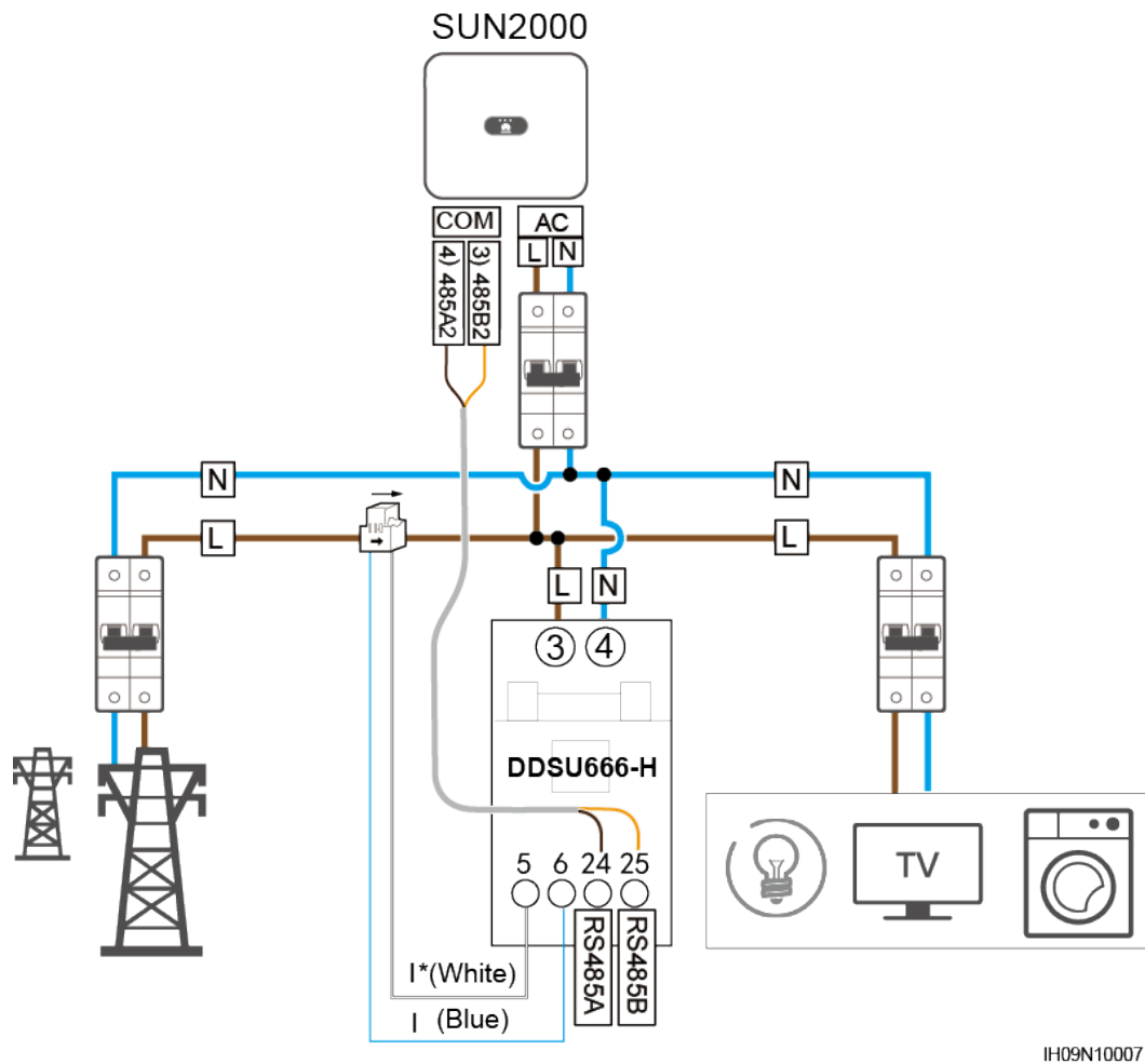
Figura 5-29 Conexión de los cables al contador de potencia DDSU666-H
