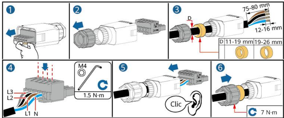
Figura 5-7 Cable de cuatro conductores (L1, L2, L3 y N)
