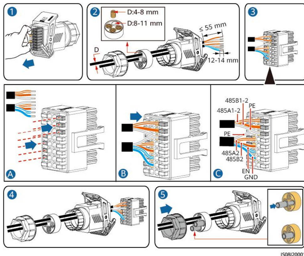
Figura 5-35 Instalación de los cables
