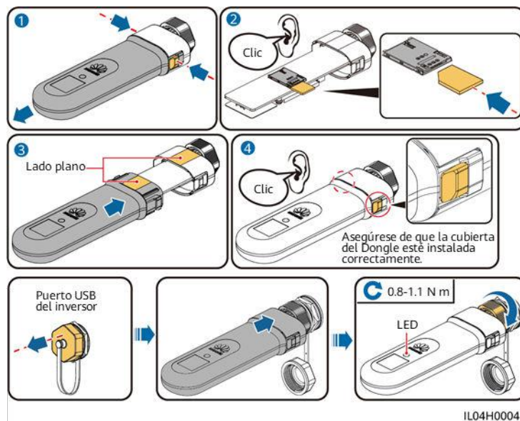
Figura 5-47 Instalación del Smart Dongle 4G (SDongleB-06)
