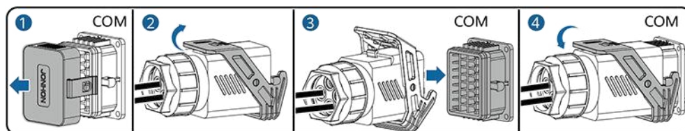
Figura 5-44 Fijación del conector del cable de señal
