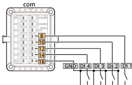
Figura 5-39 Conexión de cables
