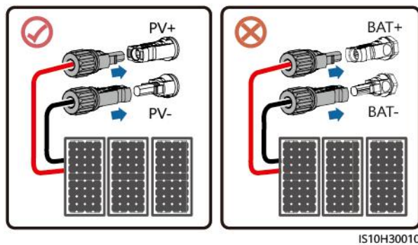
Figura 5-12 Conexión
