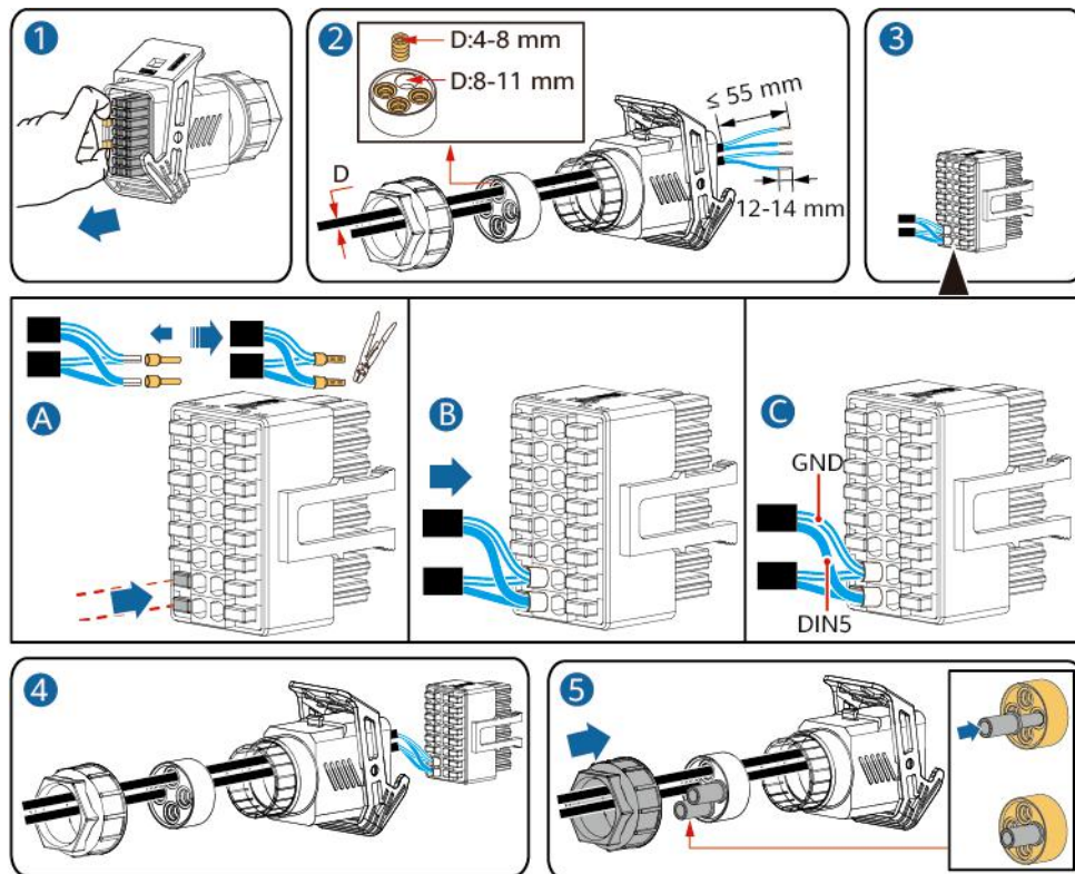
Figura 5-43 Instalación de los cables
