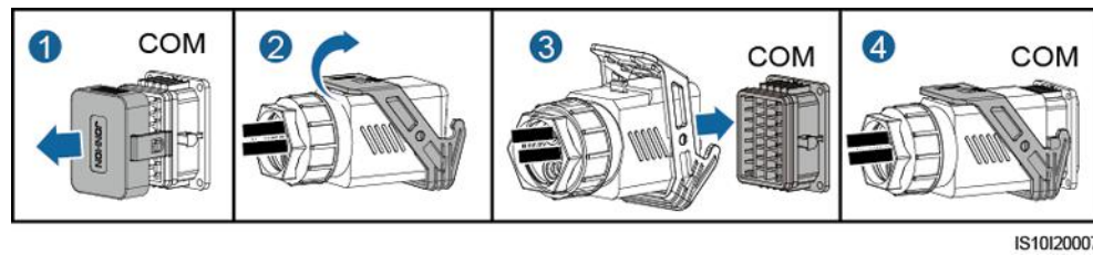
Figura 5-34 Fijación del conector del cable de señal
