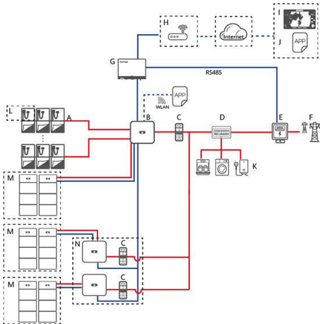
Figura 2-4 Conexión en red del SmartLogger (los componentes opcionales están encerrados en cuadros de rayas pequeñas)
