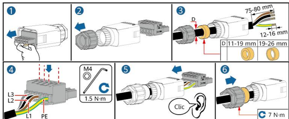
Figura 5-6 Cable de cuatro conductores (L1, L2, L3 y PE)
