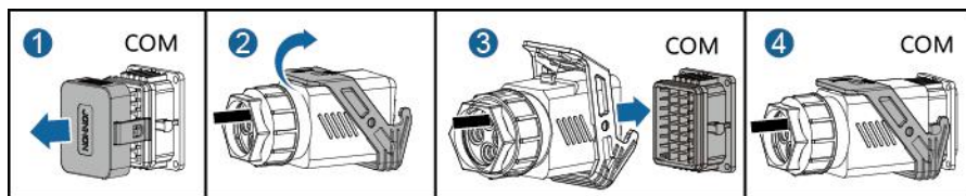
Figura 5-41 Cómo ajustar el conector del cable de señal
