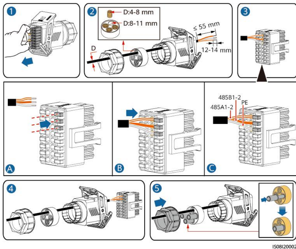
Figura 5-31 Instalación del cable
