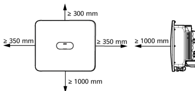
Figura 4-2 Espacio libre
