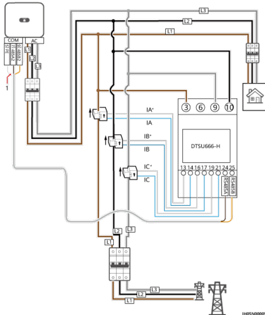
Figura 5-22 Conexión de cables trifásicos y trifilares del DTSU666-H (conexión en red del Smart Dongle)
