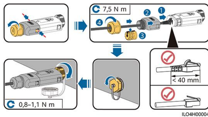
Figura 5-45 Instalación de un Smart Dongle WLAN-FE (comunicación FE)
