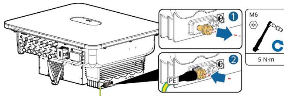
Figura 5-3 Conexión del cable de tierra
