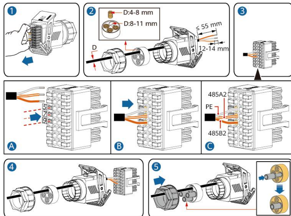
Figura 5-29 Cómo instalar el cable
