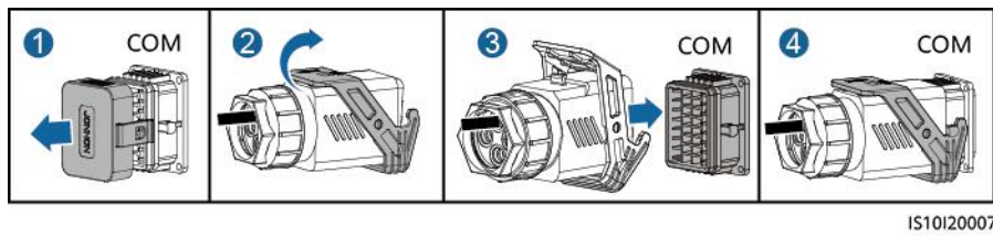
Figura 5-32 Fijación del conector del cable de señal
