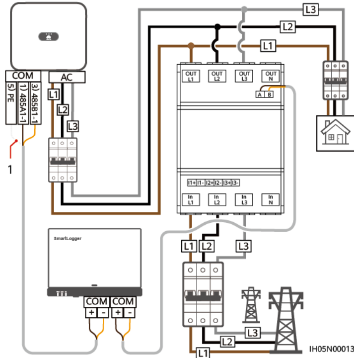
Figura 5-27 Conexión directa, trifásica y trifilar (conexión en red del SmartLogger)
