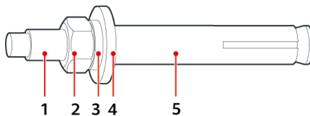
Figura 4-6 Estructura de un tornillo de expansión M6
