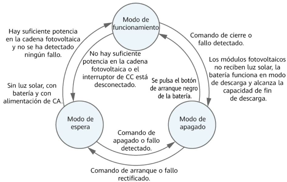
Figura 2-9 modos de operación
