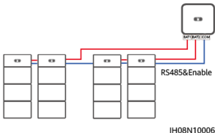
Figura 2-6 Conexión del inversor a cuatro baterías
