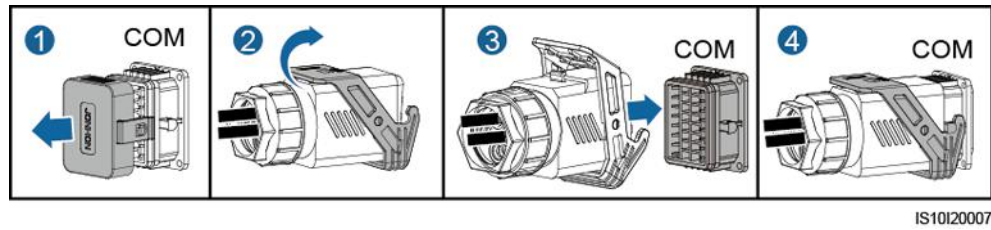
Figura 5-36 Fijación del conector del cable de señal
