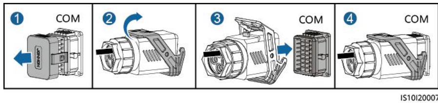
Figura 5-38 Cómo ajustar el conector del cable de señal
