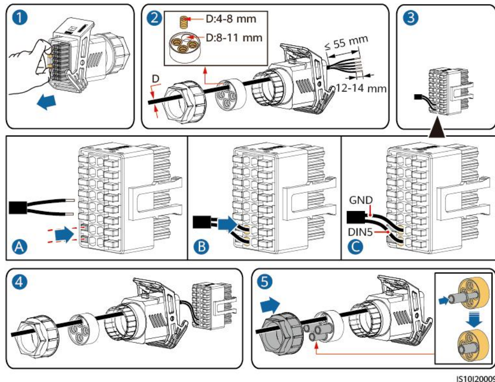
Figura 5-37 Cómo instalar el cable
