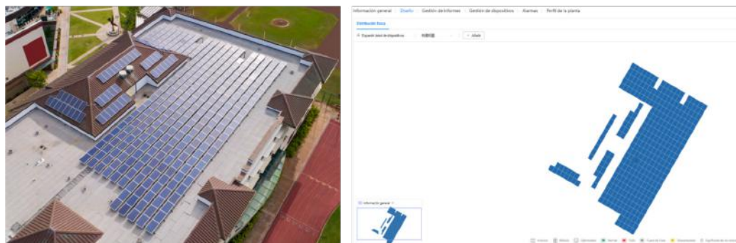
Figura 7-6 Visualización de una distribución física en el FusionSolar SmartPVMS
