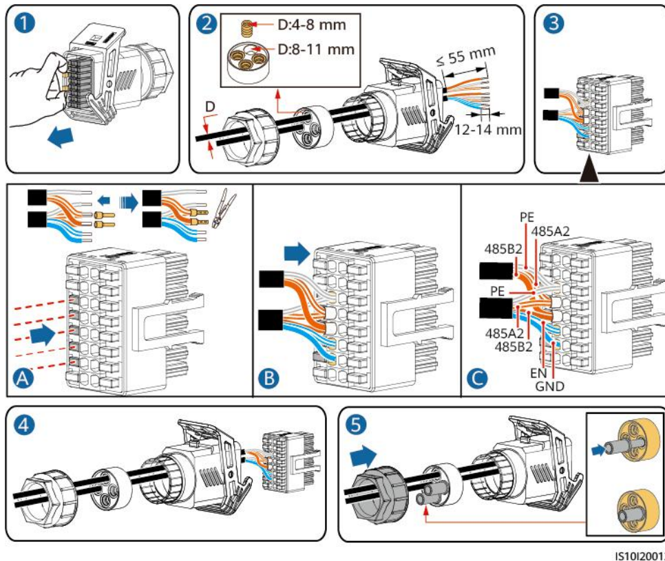
Figura 5-33 Instalación de los cables
