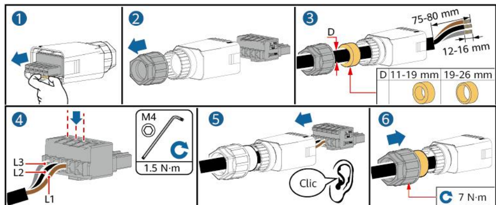
Figura 5-5 Cable de tres conductores (L1, L2 y L3)
