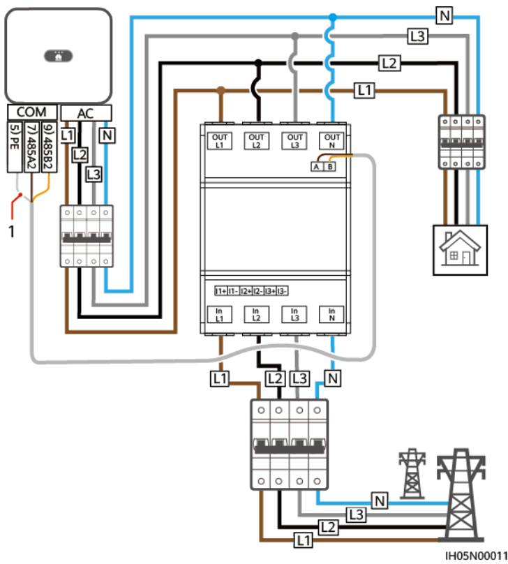
Figura 5-26 Conexión directa y trifásica de cuatro hilos (conexión en red del Smart Dongle)
