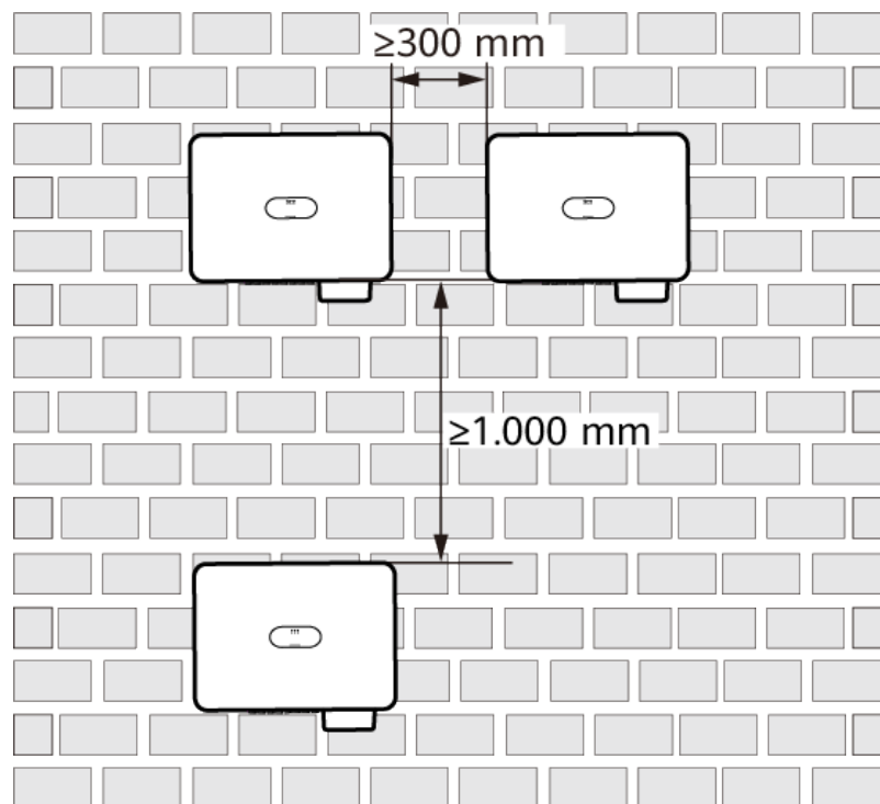
Figura 4-7 Instalación apilada sobre una pared (no recomendada)
