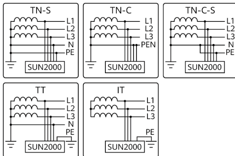
Figura 2-4 Sistemas de puesta a tierra
