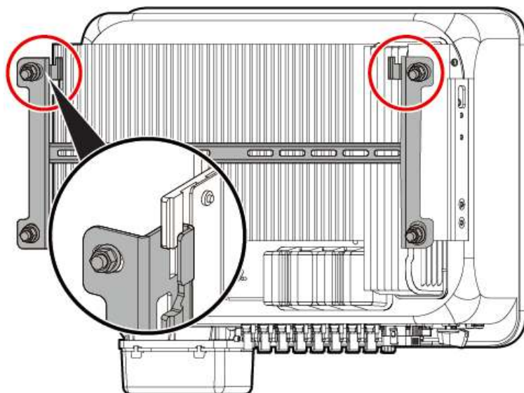
Figura 4-13 Instalación del inversor
