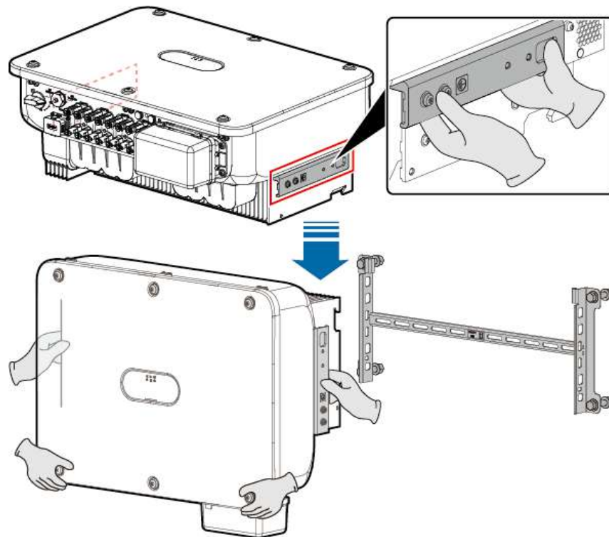
Figura 4-10 Traslado del inversor
