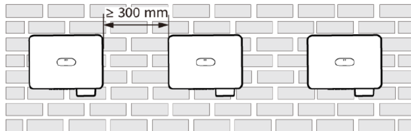
Figura 4-4 Instalación horizontal (recomendada)
