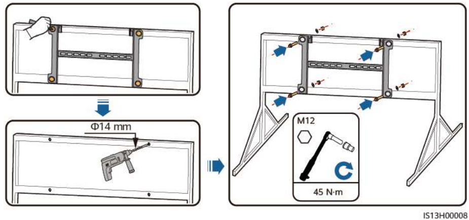
Figura 4-15 Fijación del soporte de montaje
