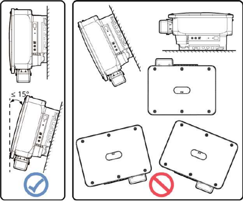
Figura 4-9 Ángulo de instalación
