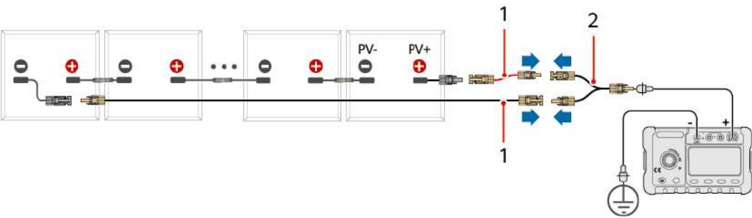
Figura 5-19 Medición de la resistencia de aislamiento del cable de extensión
