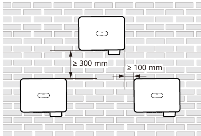
Figura 4-5 Instalación triangular en dos capas (recomendada)
