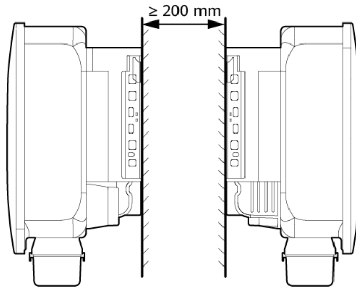
Figura 4-8 Instalación espalda con espalda sobre una pared (no recomendada)
