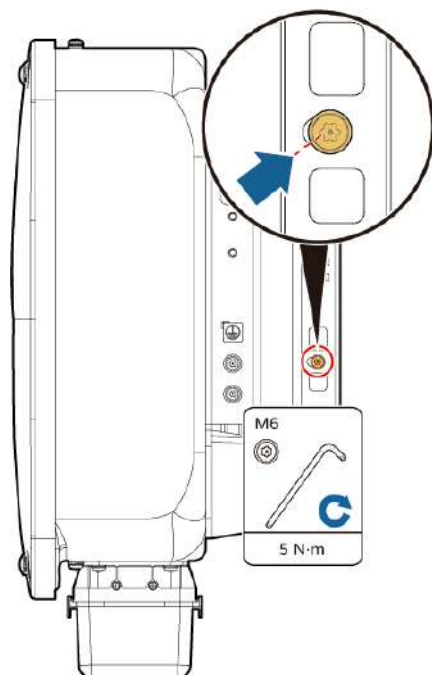
Figura 4-14 Cómo apretar los tornillos
