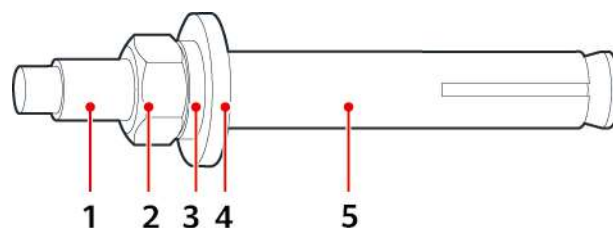
Figura 4-11 Estructura de un tornillo de expansión
