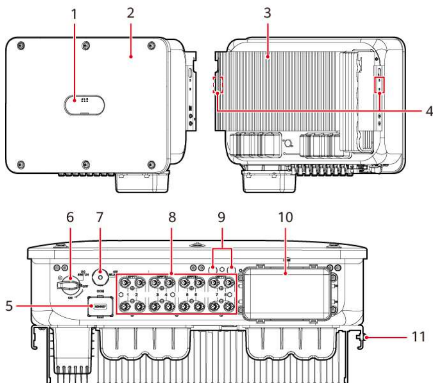
Figura 2-5 Aspecto
