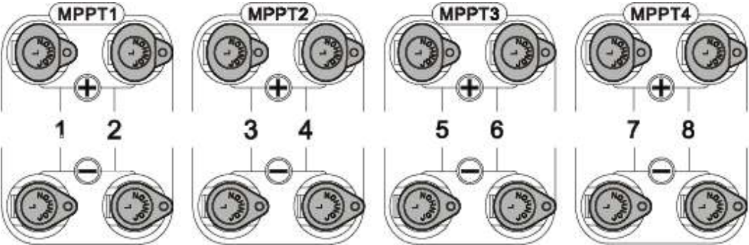
Figura 5-12 Bornes de entrada de CC
