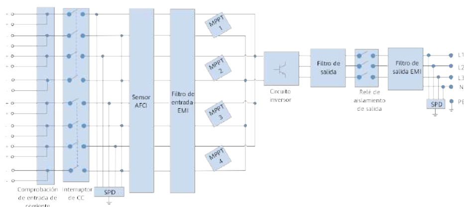
Figura 2-7 Diagrama esquemático
