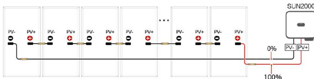
Figura 8-3 Definición del porcentaje de la posición del cortocircuito (sin optimizadores configurados)
