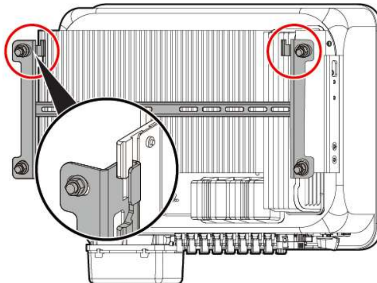
Figura 4-16 Instalación del inversor
