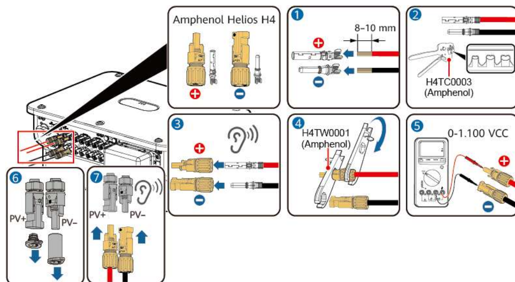
Figura 5-21 Montaje de los conectores de CC
