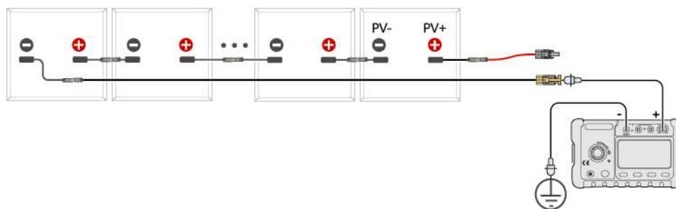
Figura 5-17 Medición de la resistencia de aislamiento de PV- para cada string FV
