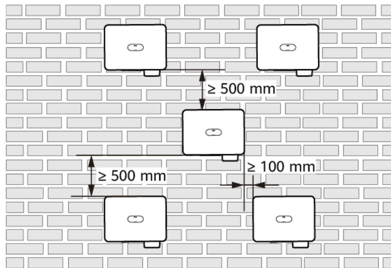
Figura 4-6 Instalación triangular en tres capas (no recomendada)
