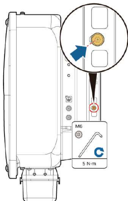
Figura 4-17 Cómo apretar las tuercas
